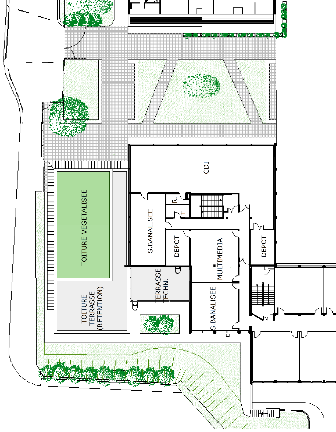
ETAT PROJETE : BAT. A – ZONE NORD : PLAN DU 1er ETAGE
