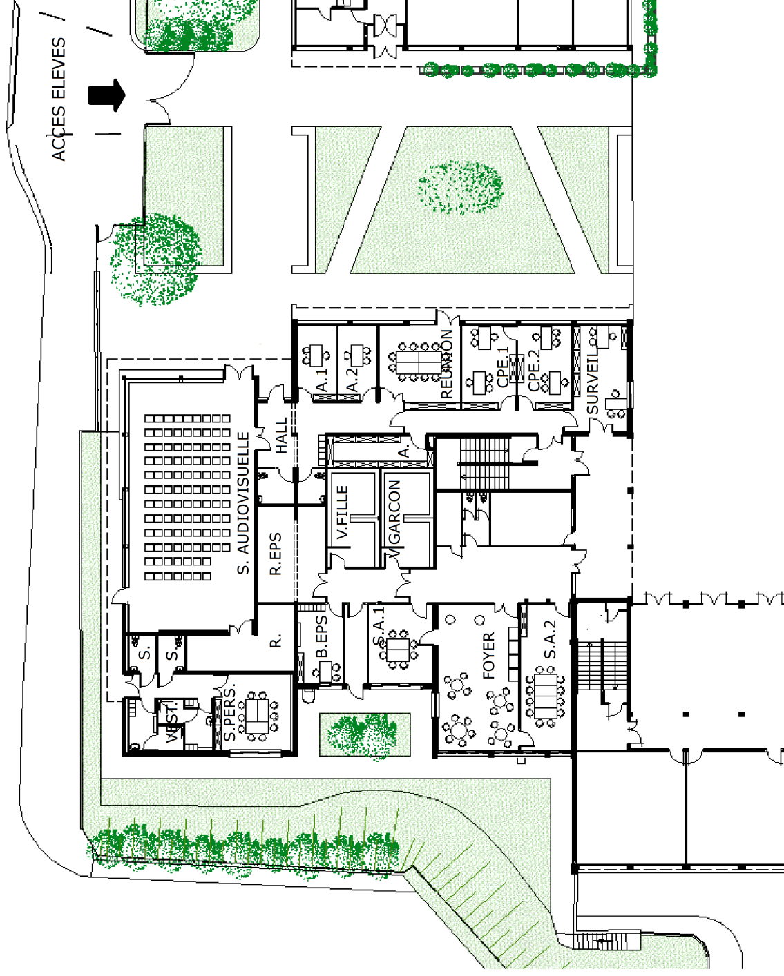
ETAT PROJETE : BAT. A – ZONE NORD : PLAN DU RDC
