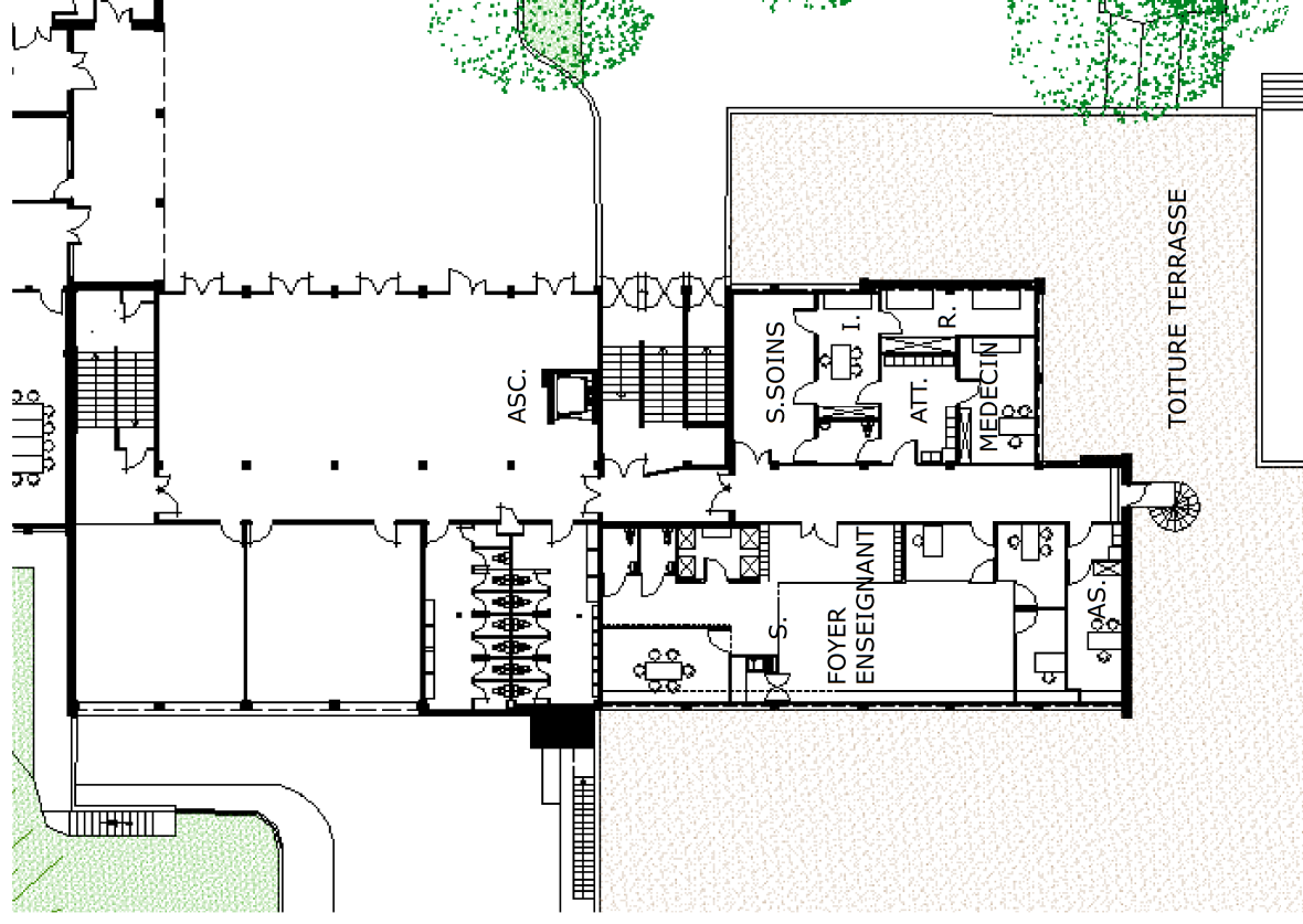
ETAT PROJETE : BAT. A – ZONE SUD : PLAN DU RDC
